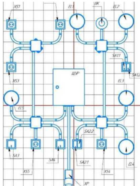
Рисунок 1 - Пример стенда для выполнения модулей 1А и 1Б.
